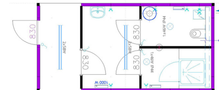
Sanitairunit
