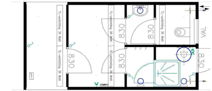
Sanitairunit
