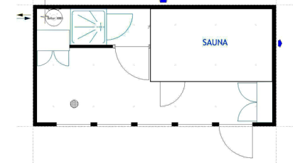
Saunaunit
